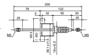
CMS5D80-1PF
