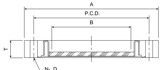
TVU-100, 150
