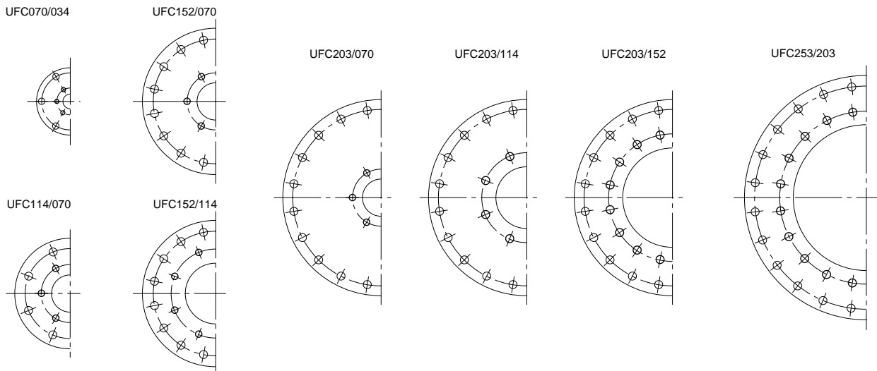
ボルト穴振り
