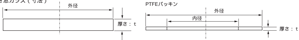
覗き窓ガラス (寸法)
