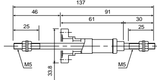
CMS5D20-1PFM
