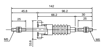
CMS5D80-1PFM
