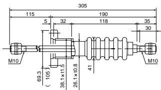
CMS10D80-1PF
