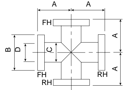
FH / 固定フランジ、RH / 回転フランジ
