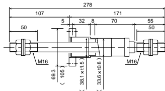
CMS16D20-1PF
