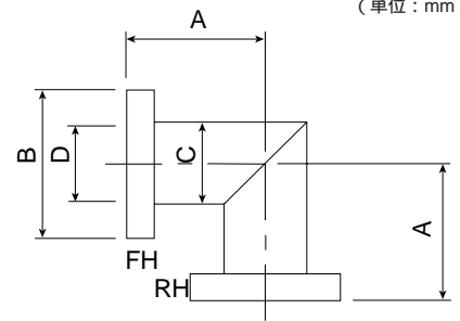
FH / 固定フランジ、RH / 回転フランジ
