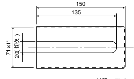
UFC070フランジ用電極カバー (オプション) 8
